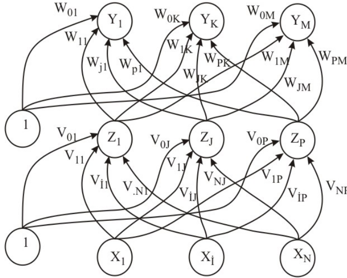
Şekil 1.2. İleri beslemeli çok katmanlı sinir ağı: x, z, y vektörleri ile V, W matrisleri
