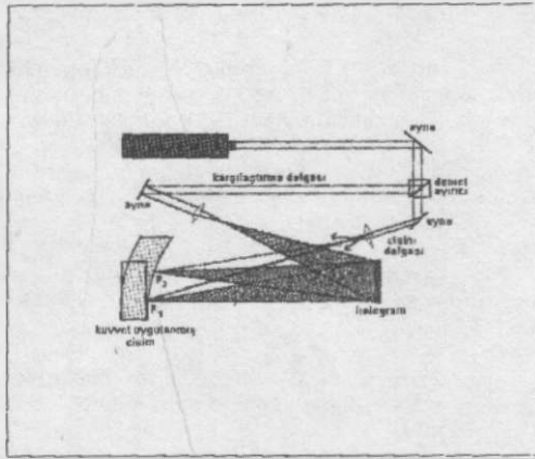
Şekil 3. Çift poz holografik kayıt yöntemi.
