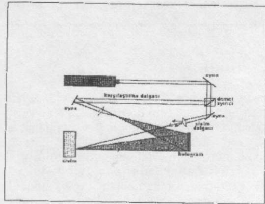
Şekil 1: Cisim görüntüsünün hologram plakasına kaydedilmesi
