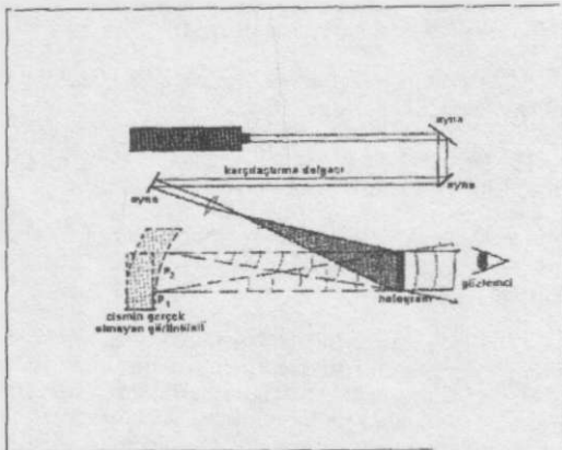
Şekil 4. Çift poz holografik görüntüün oluşturulması.
