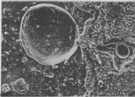
Resim 2. Aşırı nemli hazırlanmış kaşitede One Step bond- in uygulanması sırasında kırılma yüzlerinde gözlenen hava kabarcıkları ve aşırı neme bağlı düzensiz bağlanma yüzeyi.
