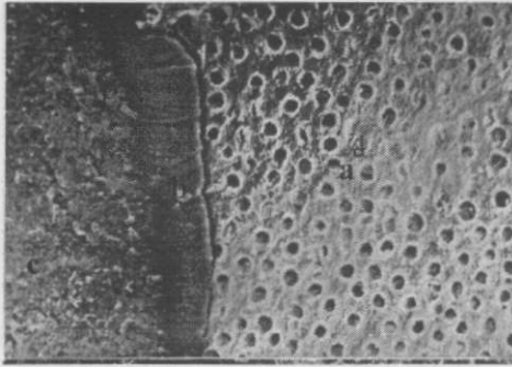
Resim 1. One step grubuna ait kırık tipte kırılma gösteren bir örnek. a: Dentinde kohesi ve kırılma, b: adezivde kırılma ve c: kompozit materyalde kırılma.
