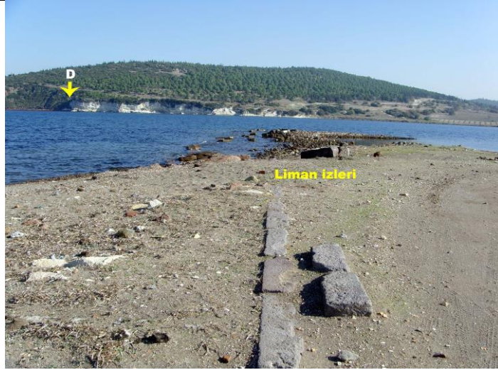
Şekil 2. Myrina limanı kalıntıları ve andezit-marn dokunağı (D)
