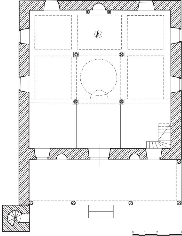
Şekil 1- Irlamaz Köyü Camii. Plan.
