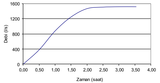
Çizelge 10. Akdoğan Havzası ortalama birim hidrografi (BH 60 ordinat değerleri ve S 60 hidrografi
