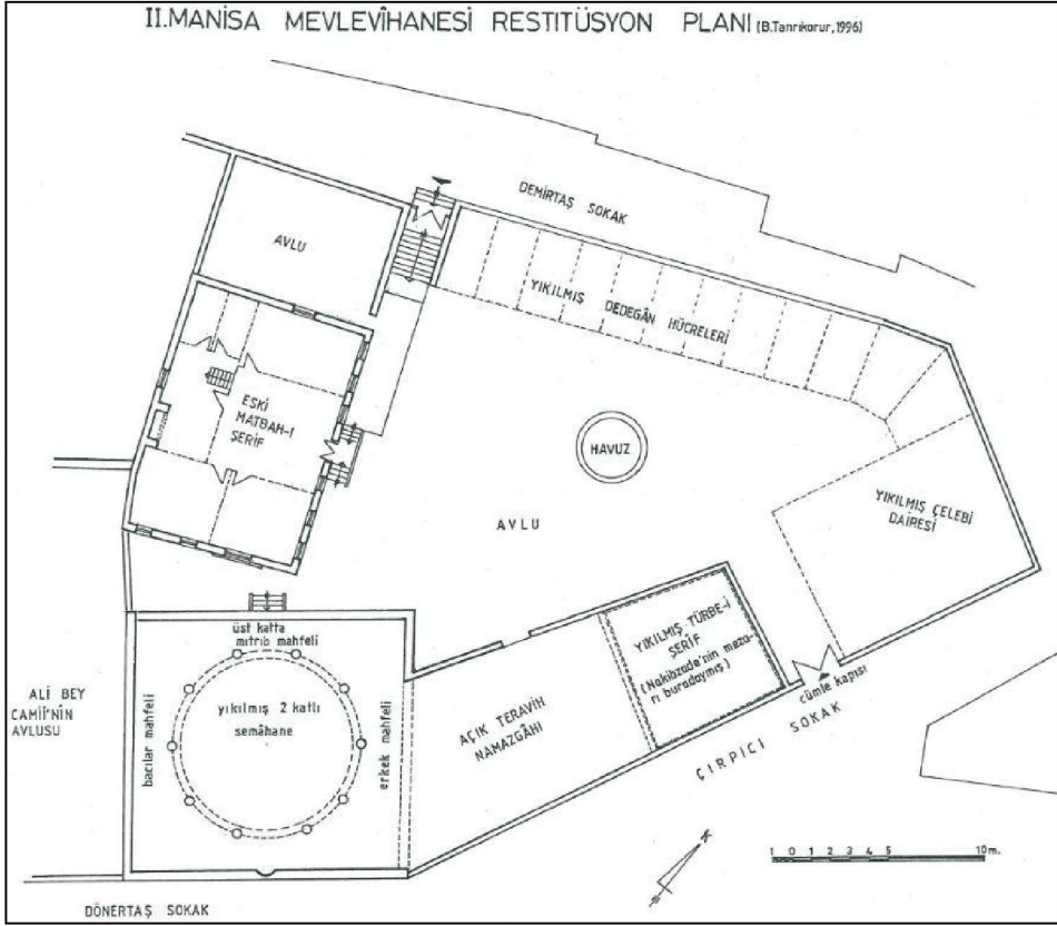
Çizim 2: İkinci Manisa Mevlevihanesi Restitüsyon Planı (B. Tanrıkorur, 1996) 158
