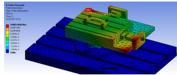
Şekil 7. Toplam deformasyon (birim şekil değişimi)
