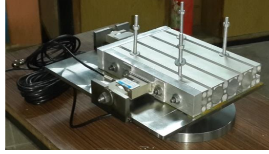
Şekil 2. Yük hücrelerinin çeşitli bağlama aparatlarıyla bir tablaya bağlanmasıyla oluşan dinamometre tasarımı
