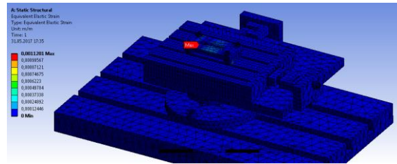
Şekil 8. Elastik gerilme (birim yerdeğiştirme)
