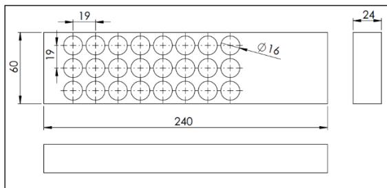
Fig. 1. Test sample (Özkul 2012)
