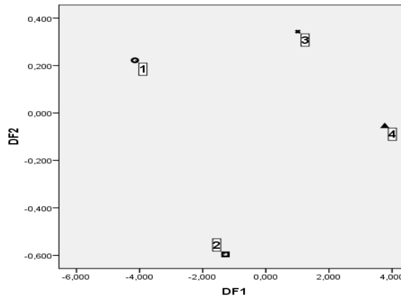
Şekil 1: Dokuz Yordayıcı Değişkenden Elde Edilen 2 Ayırma Fonksiyonunda, 4 Grubun Ayırma Fonksiyonu Puan Ortalamaları (Centroid) Grafiği (1- Evlilik Uyumu Düşük Kadın, 2- Evlilik Uyumu Yüksek Kadın, 3- Evlilik Uyumu Düşük Erkek, 4- Evlilik Uyumu Yüksek Erkek)
