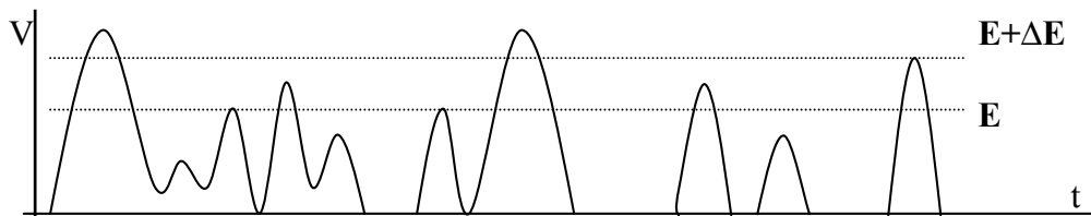
Şekil 2. , na yükselteç çıkışındaki pulslar ve seçilen E, E+ΔE seviyeleri
