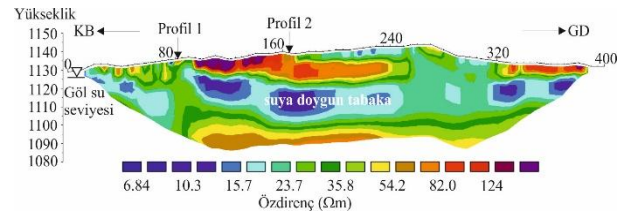
Şekil 3: Profil 3 için 2-B özdirenç kesit.
