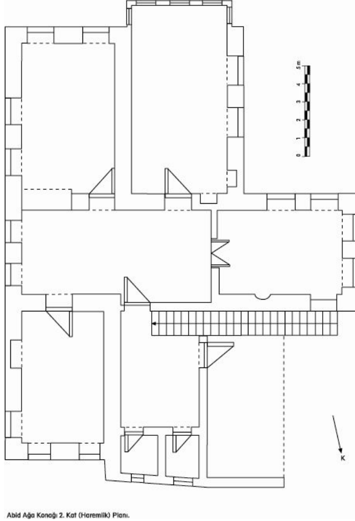
Abid Ağa Konağı 2. Kat (Haremlik) Planı.
