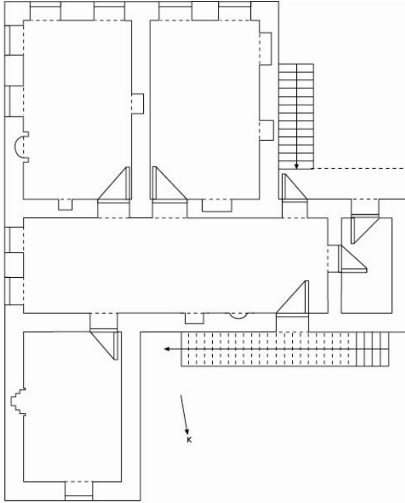
Abid Ağa Konağı 1. Kat (Selamlık) Planı.
