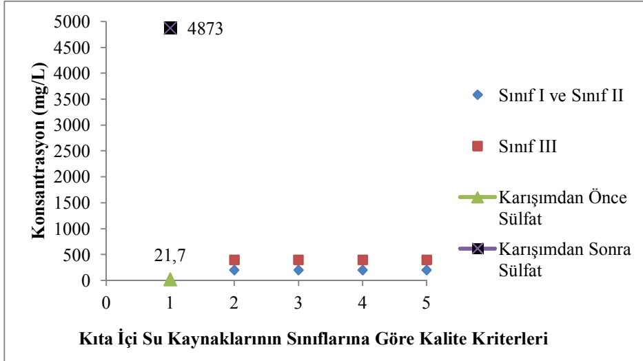
Şekil 5. Maden çayının sülfat konsantrasyonu değişimi.
