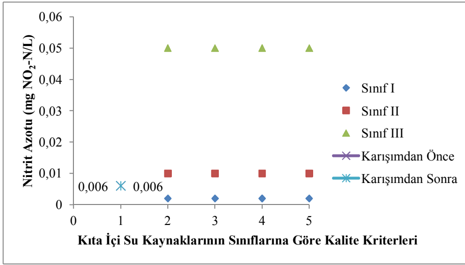
Şekil 7. Maden çayının nitrit azot konsantrasyonu değişimi.
