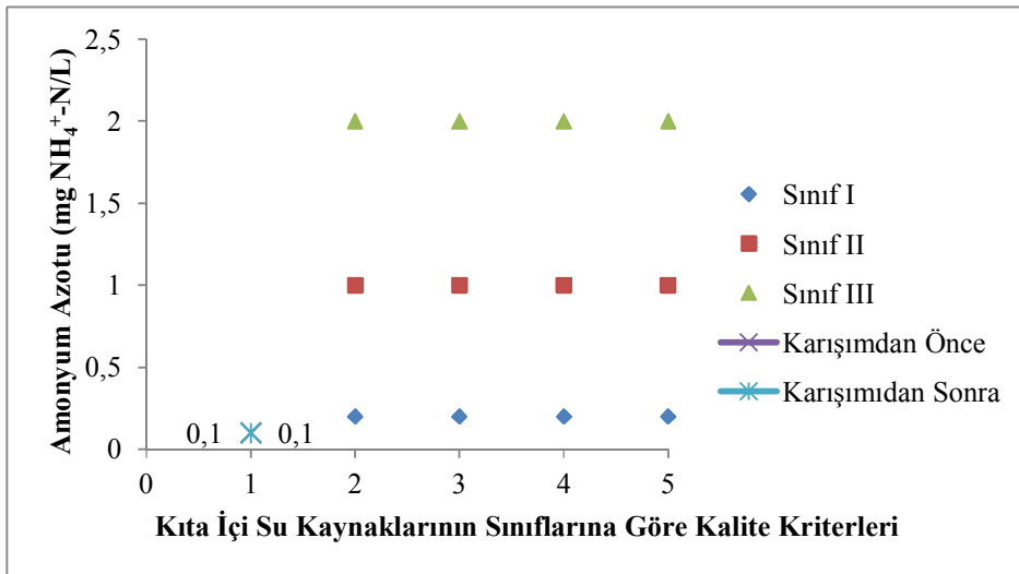
Şekil 6. Maden çayının amonyum azot konsantrasyonu değişimi.
