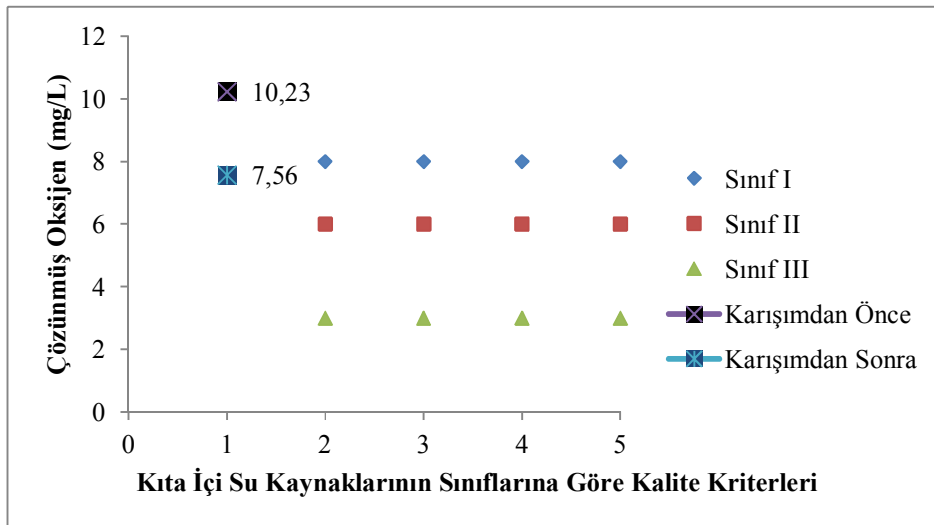
Şekil 3. Maden çayının ÇO konsantrasyonunun değişimi.
