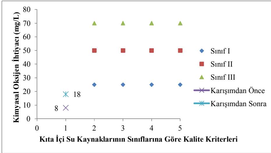
Şekil 4. Maden çayının KOİ konsantrasyonunun değişimi
