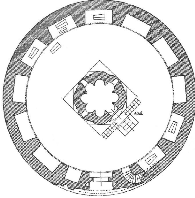
Şekil 4- Tercan Mama Hatun Türbesi, Plan (S. K. Yetkin'den)
