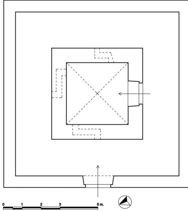
Şekil 2- Tarsus Duatepe Türbesi, Plan (H. Sibel Ünalın).
