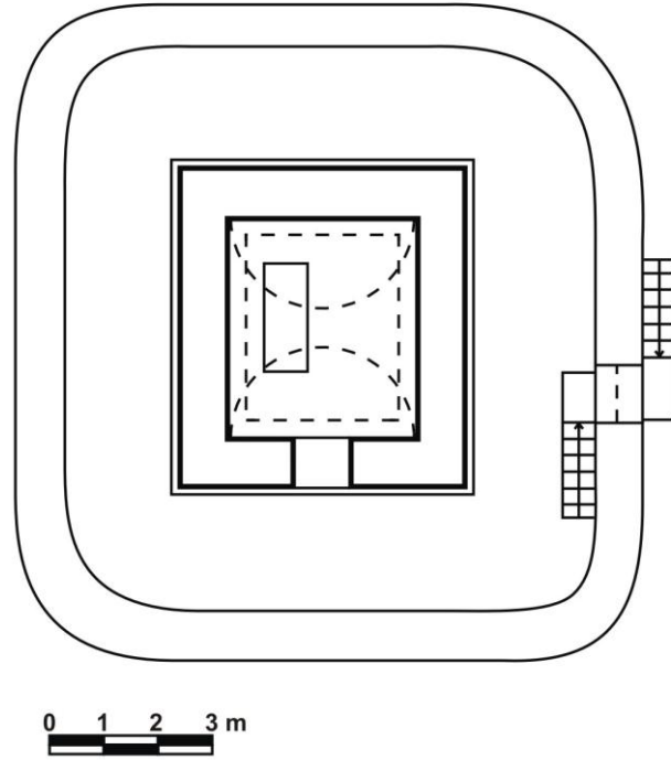
Şekil 3- Kayseri-Talas-Sakaltutan Köyü Mikdat Dede Türbesi, Plan (F. İlder'den)
