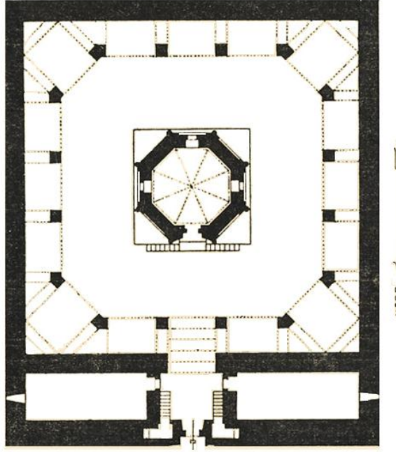
Şekil 5- Kayseri Köşk Medrese, Plan (A. Gabriel'den)
