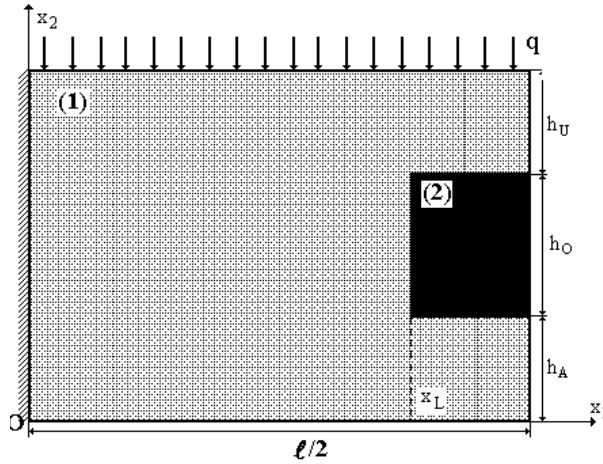
Şekil 1. Ele alınan şerit-levhannın geometrisi
