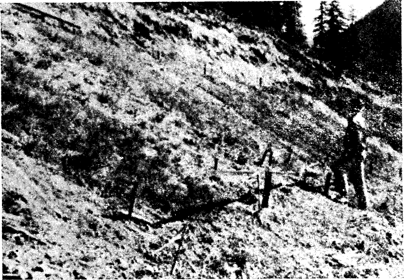
Şekil 7. Tohumlamadan 7 ay sonraki dolduru şevi deneme plotlarının görünüşü. Şevin profilini çıkarmak maksadiyle faydalanılan tel halat U demirleri arasında gerilmiştir.
