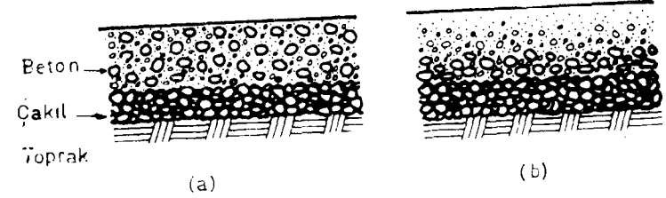
Resim 4. İyi (a) ve kötü (b) beton kaplama enine kesitleri.
