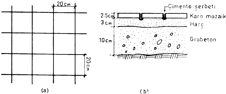
Resim 9. Karomozaik kaplama; (a) üstten görünüş, (b) kesit.
