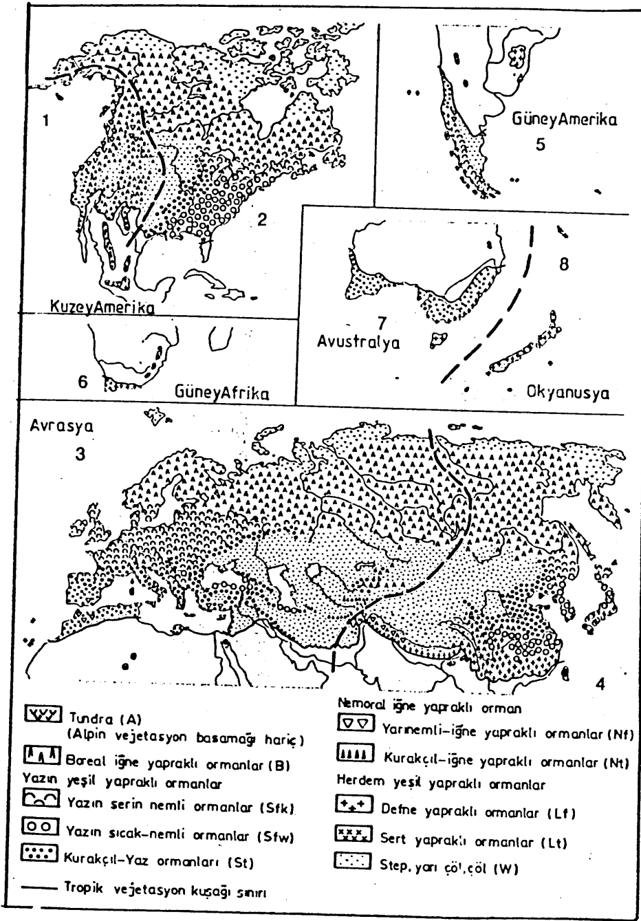
Şekil 1: Zonal vejetasyon tipleri (SCHROEDER 1976)
