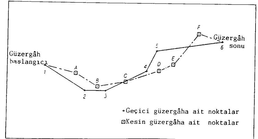
Şekil 9 : Geçici Güzergâhın Üzerine İşaretlenen Kesin Güzergâh
