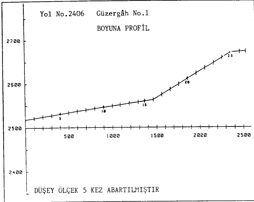
Şekil 10 : ROUTES Programı İle Elde Edilen Güzergâh Profili
