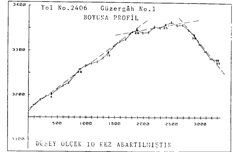
Şekil 3 : Mevcut Bir Yol Profilinden Büyük Eğim Farklarının Belirlenmesi
