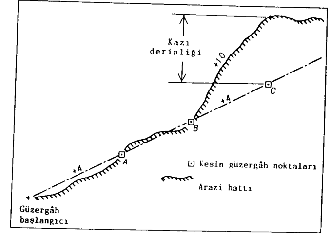
Şekil 8 : Eğim Hattında Bir Arazi Noktası Bulunmadığında Kazı Derinliğinin Bulunması
