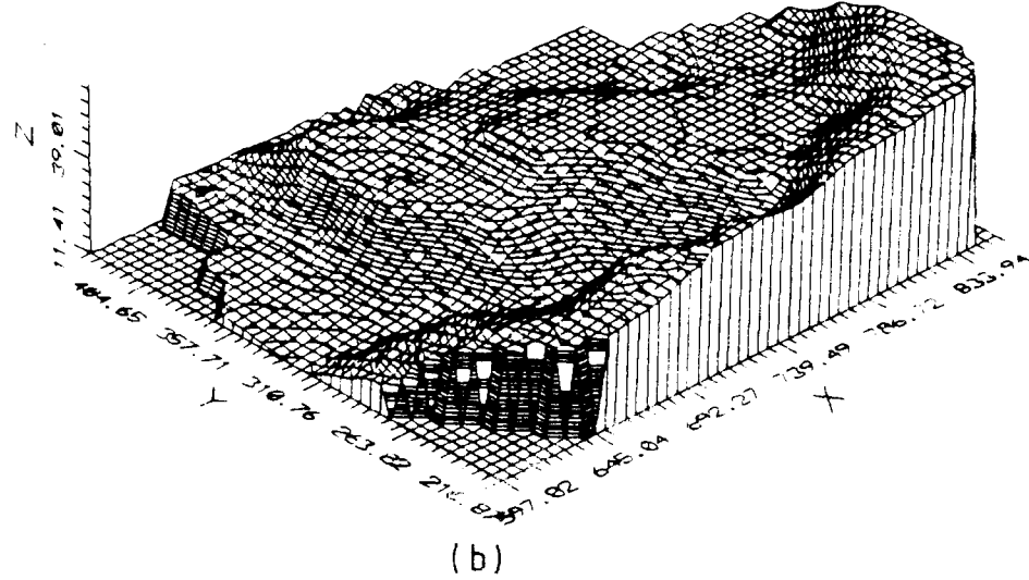
Şekil 3 : Uygulama Sahasının (Dolgu Yapılmadan Önce) 176 Adet Dayanak Noktasından Elde Edilen Perspektif Görünümü
