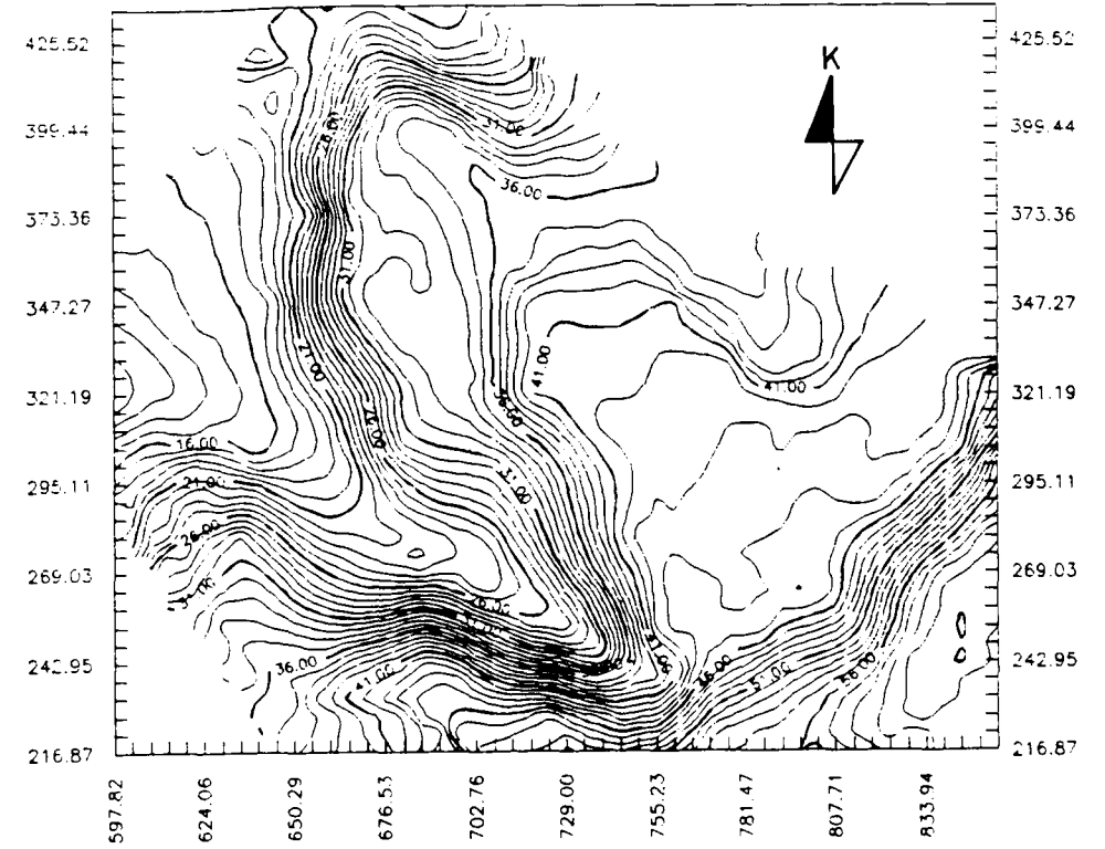
Şekil 2 : Uygulama Sahasının (Dolgu Yapılmadan Önce) 176 Adet Dayanak Noktasından Elde Edilen Topoğrafik Haritası
