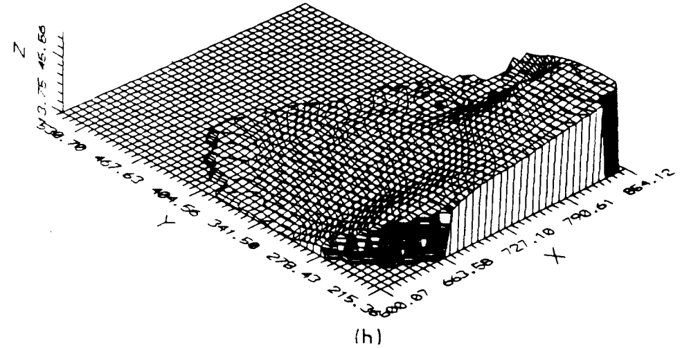
Şekil 6 : Uygulama Sahasının (Dolgu Yapıldıktan Sonra) 102 Adet Dayanak Noktasından Elde Edilen Perspektif Görünümleri
