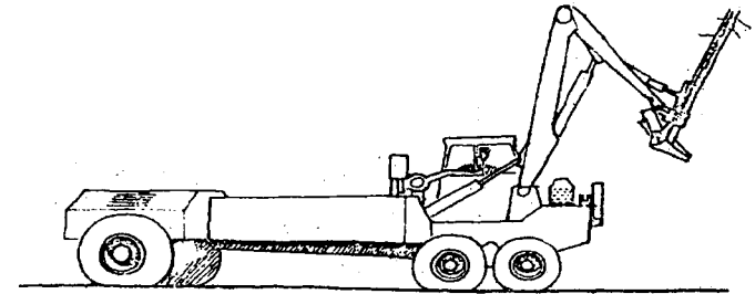
Devirme-dal alma ve tomruklama makinesi (prosesör)
