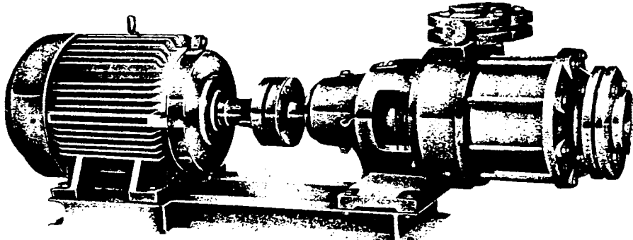
Şekil 2: Motor - Pompa
