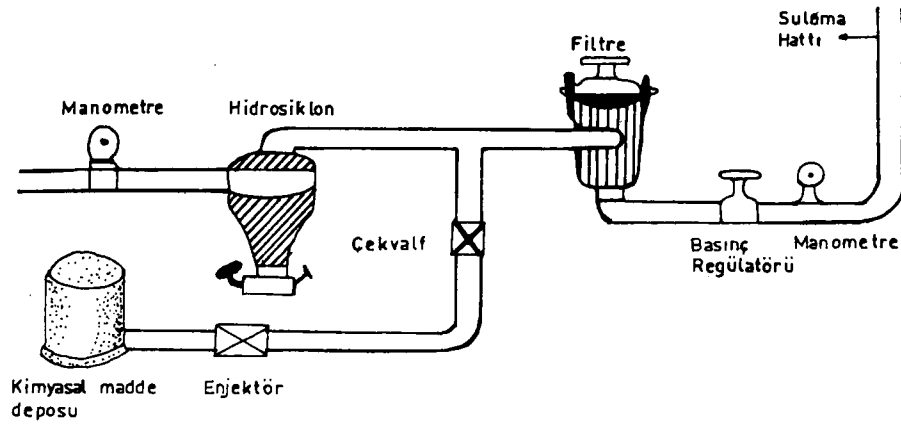
Şekil 6: Yardımcı elemanlar
