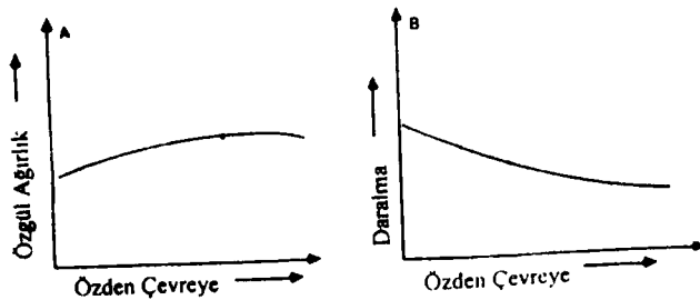
Şekil 2: Yapraklı ağaçlarda özgül ağırlık ve daralma değerlerinin özden çevreye doğru değişimi (MAEGLIN 1987).
