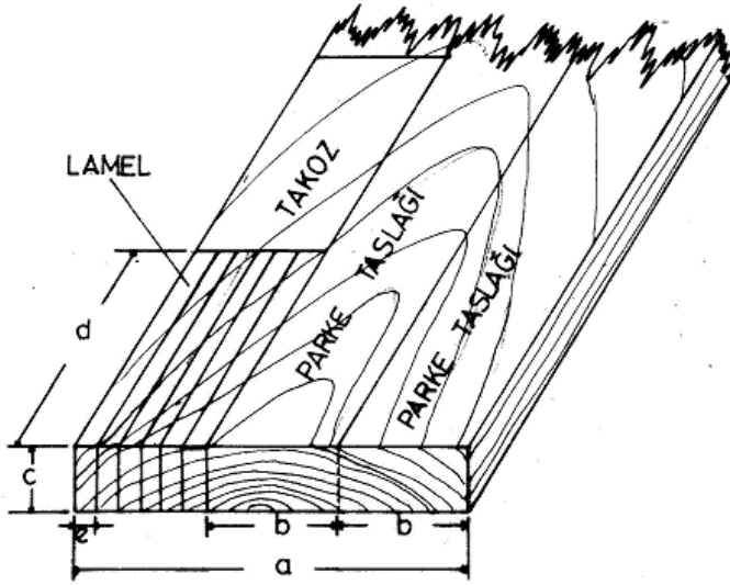
Şekil 2. Parkelik kereste ve bu keresteden klasik mozaik parke taşı, takoz ve lamellerin elde edilmesi. a parkelik kereste genişliği, b klasik mozaik parke taşı genişliği veya takoz genişliği, c kereste kalınlığı veya takoz kalınlığı veya lamel genişliği, d takoz uzunluğu veya lamel uzunluğu, e lamel kalınlığı.
