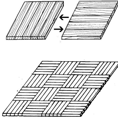
Şekil 3. İki lamel karesinin (veya kare desenin) lifleri birbirine dik olacak şekilde birleştirilmesi ve lamel karelerinden oluşmuş mozaik parke paneli (veya mozaik parke döşeme ünitesi).
