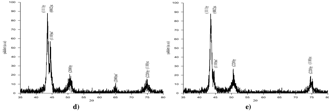
Şekil 5. a)Austenite yapıda,b) 700 °C’de, c) 800 °C’de, d) 900 °C’de ve e) 1000 °C’de ısıtım işlem uygulanmış Fe -%18,79Mn-%4,53Ni alaşımının X-ışını kırınım deseni
