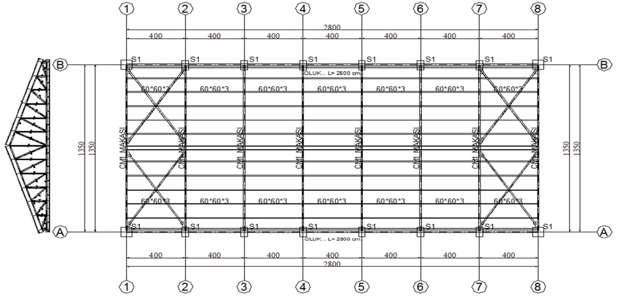
ÇATI APLİKASYON PLANI Ö: 1/100
