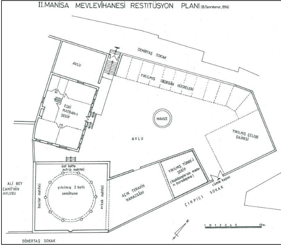
Çizim 2: İkinci Manisa Mevlevîhanesi Restitüsyon Planı (B. Tanrıkorur, 1996) 158
