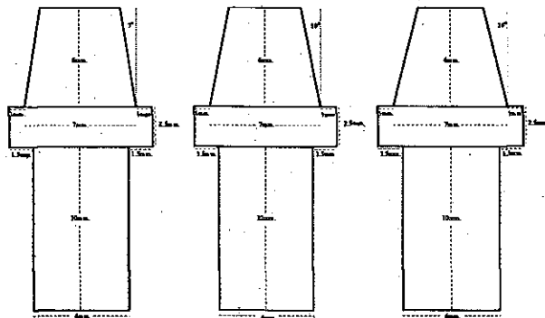
Şekil 2. Hazırlanan dişlerin boyutları
