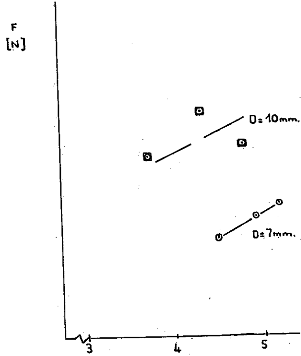
Grafik 3. Tutucu kuvvetin üst yüzey, yan yüzey ve toplam yüzey alan ile değişimi.
