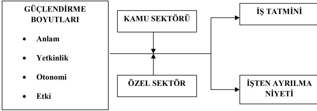
Şekil 1. Araştırmanın Modeli
