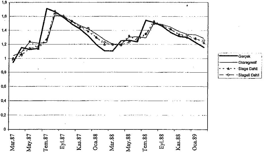
Şekil 9: Reel verilerle hesaplanan tüç modelin 1987-1988 yılları arasındaki tahmini değerleri ve gerçek değerleri (indeks)
