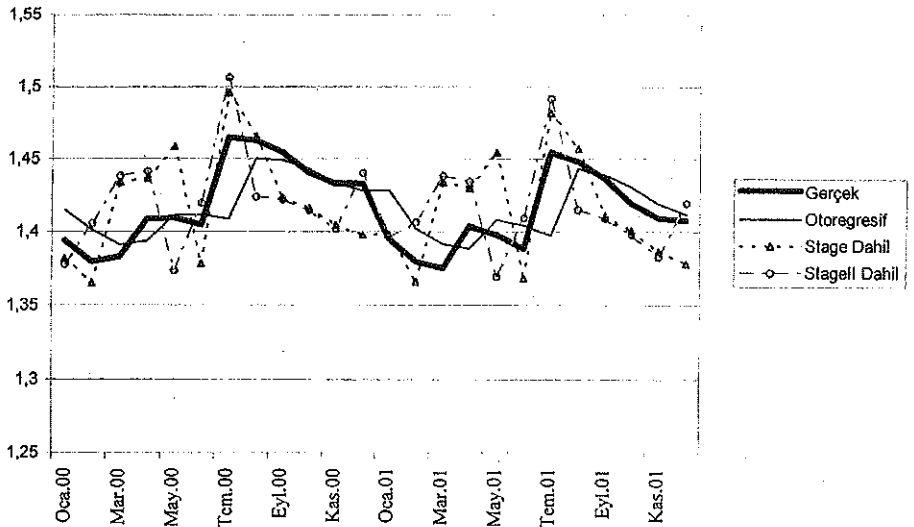
Şekil 10: Reel verilerle hesaplanan tüç modelin 2000-2001 yılları arasındaki tahmini değerleri ve gerçek değerleri (indeks)
