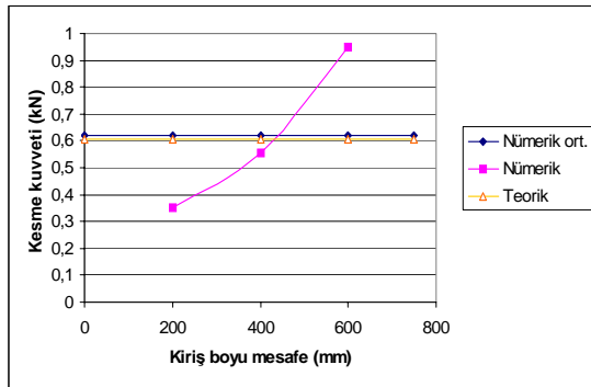
Şekil 6. Kiriş boyunca basınç bölgesindeki ara yüz kesme kuvvetleri (Model 1).
