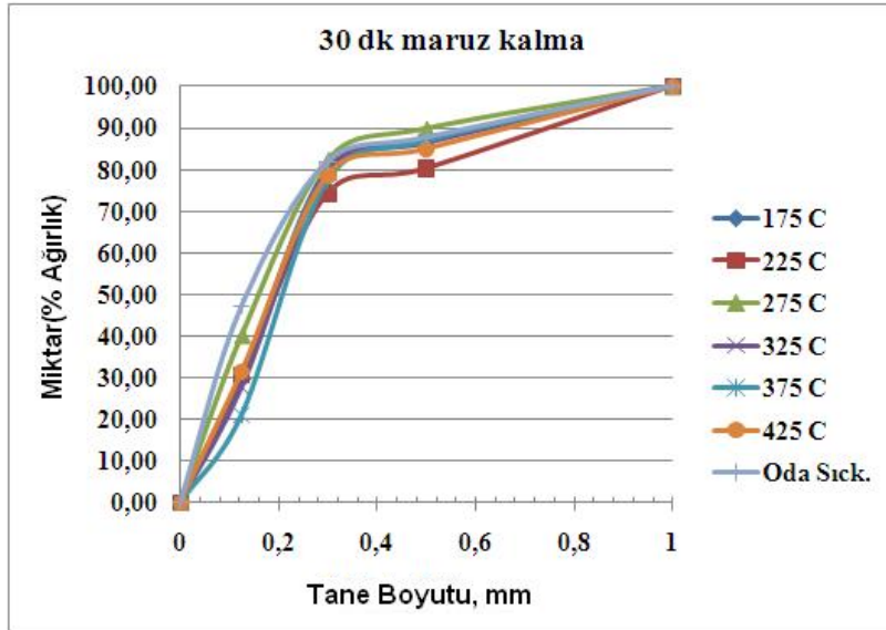
Şekil 12: Konvs. ısıtma, 30 dk maruz kalma
