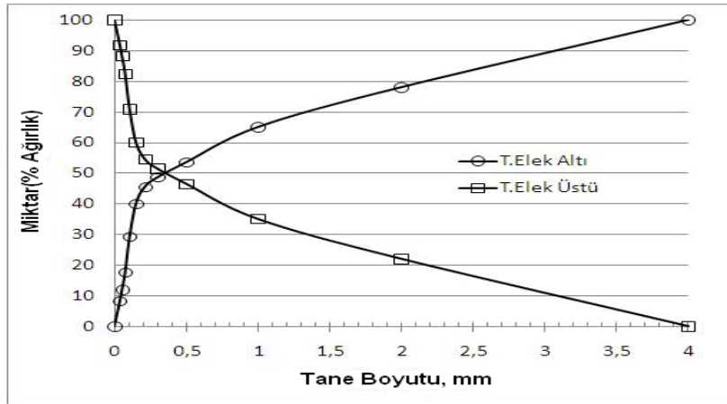
Şekil 7: Öğütme deneyleri öncesinde numunenin kümülatif elek eğrileri
