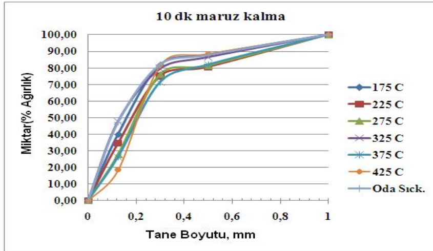
Şekil 10: Konvs. ısıtma, 10 dk maruz kalma
