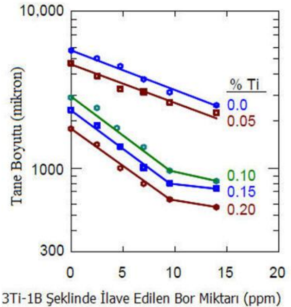
Şekil 7. Alüminyum 319 alaşımında tane inceltme sonuçları [9].
