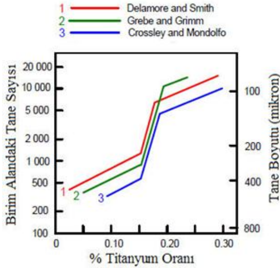
Şekil 5. % 99,7 safiyette alüminyumda titanyum ilavesi ile tane inceltme sonuçları [6].
