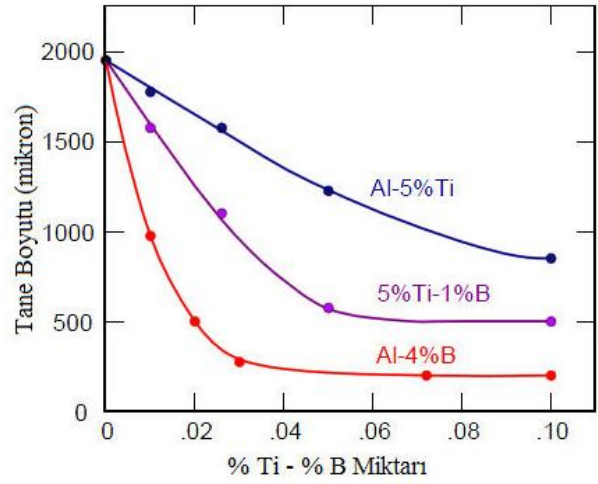
Şekil 6. A356 alüminyum alaşımında üç farklı mastır alaşımı ile tane inceltme sonuçları [7].
