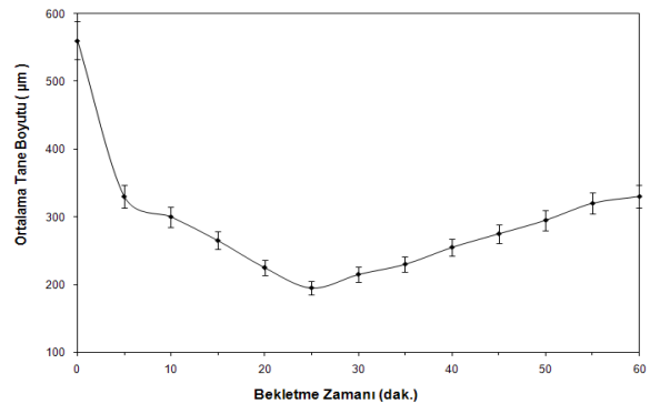
Şekil: 4. ETİAL 160 primer alaşımına katılan Al5Ti1B master alaşımının bekleme zamanına göre tane boyutu değişimi [5].
