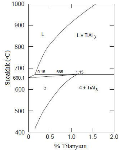
Şekil: 2. Al-Ti Faz diyagramının alüminyum tarafı [2].
