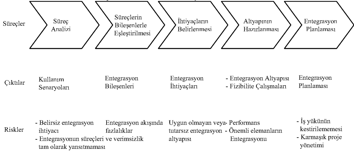
ŞEKİL 6: EIM Yaklaşımı
