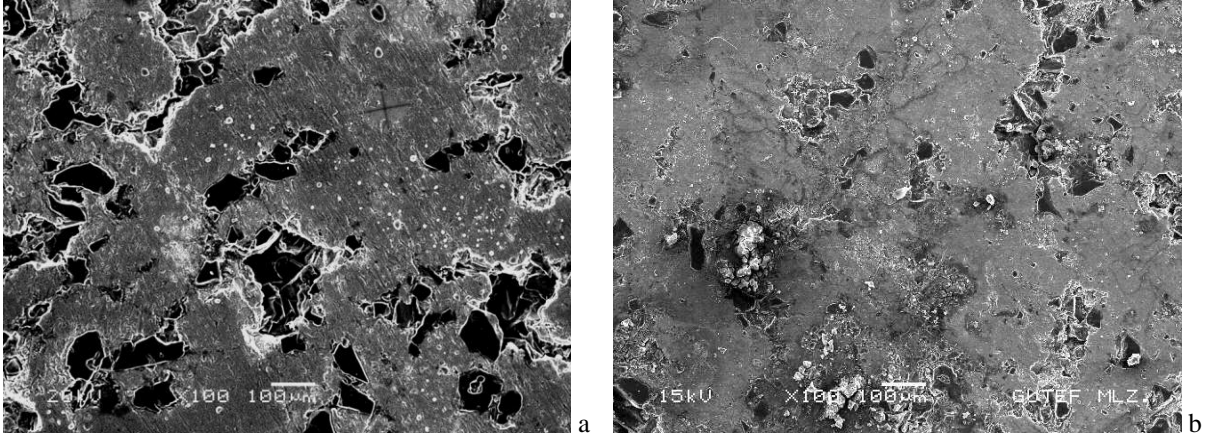
Şekil 8. % 20 B 4 C takviye sonrası 24 h yaşlanma (24 h aged after 20% B 4 C Reinforced)
