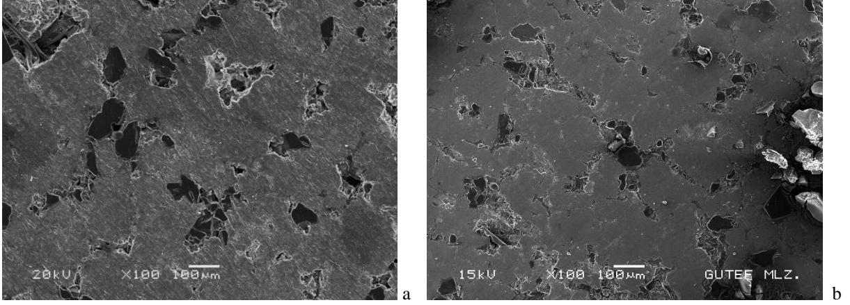
Şekil 7. % 10 B 4 C takviyeli (10% B 4 C-Reinforced)
