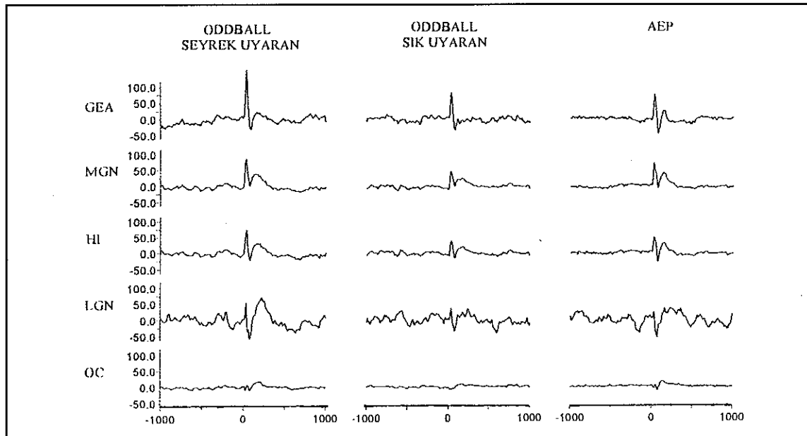
Şekil 2. Bir kedinin GEA, MGN, HI, LGN ve OC işitsel oddball paradigması ile sık ve seyrek uyarılara karşı kaydedilen yanıtlar ve standart işitsel uyarılma potansiyelleri (AEP).
