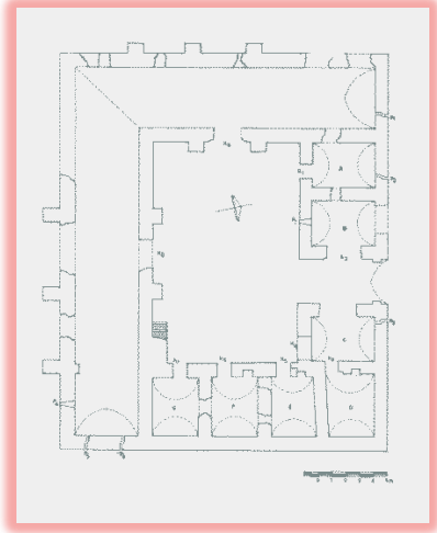
Çizim 3: Balat'ın Girişindeki Han, rölöve planı (Rölöve: Aynur Durukan-Mustafa Akpolat; Çizen: Çelik Topçu 1980)
