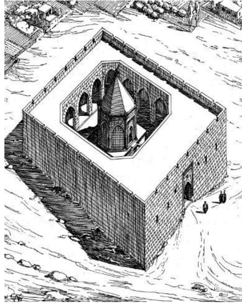
Çizim 2: Kayseri Köşk Hânkahı (Medrese) Restitüsyon Çizimi (Gabriel 1931: şekil 43)
