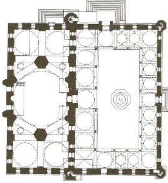
Çizim 6: Edirne Üç Şerefeli Cami planı (Goodwin 1971: şekil 93)
