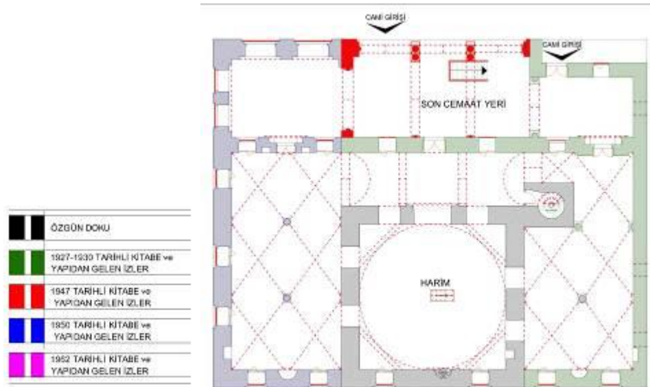
Çizim:4 - Hazro Ulu Camii Üst Kat Restitüsyon Planı Ölçek: 1/50 (Vakıflar Bölge Müdürlüğü Arşivinden).
