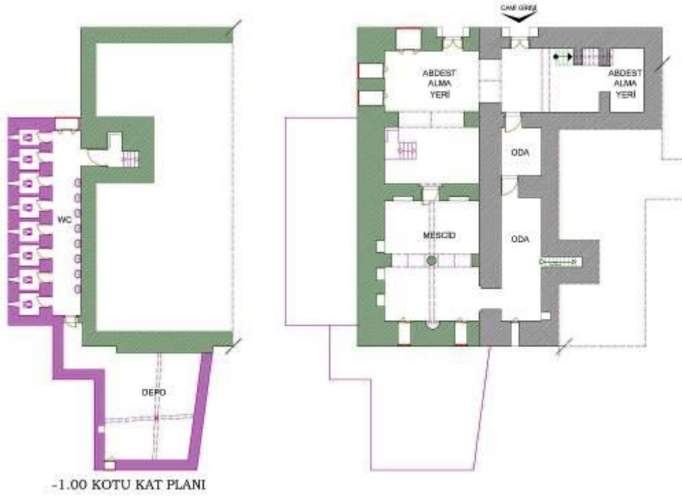
Çizim:3 - Hazro Ulu Camii'nin Zemin Kat Restitüsyon Planı Ölçek: 1/50 (Vakıflar Bölge Müdürlüğü Arşivinden).
