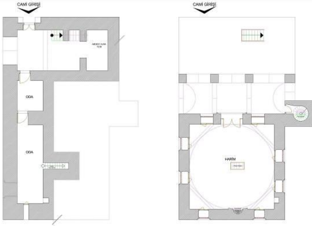
Çizim:1 - Hazro Ulu Camii'nin I. Dönem (Özgün) Zemin Kat ve Üst Kat Restitüsyon Planı Ölçek: 1/50 (Vakıflar Bölge Müdürlüğü Arşivinden).
