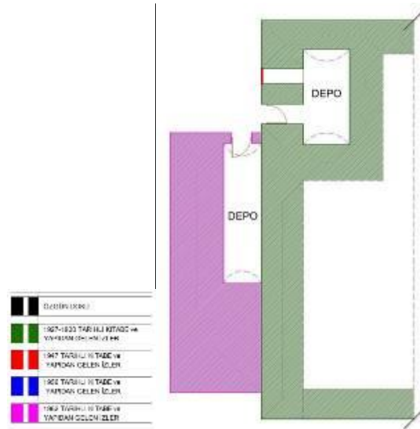
Çizim:2 - Hazro Ulu Camii'nin Bodrum Kat (-2.50 Kotu) Restitüsyon Planı Ölçek: 1/50 (Vakıflar Bölge Müdürlüğü Arşivinden).
