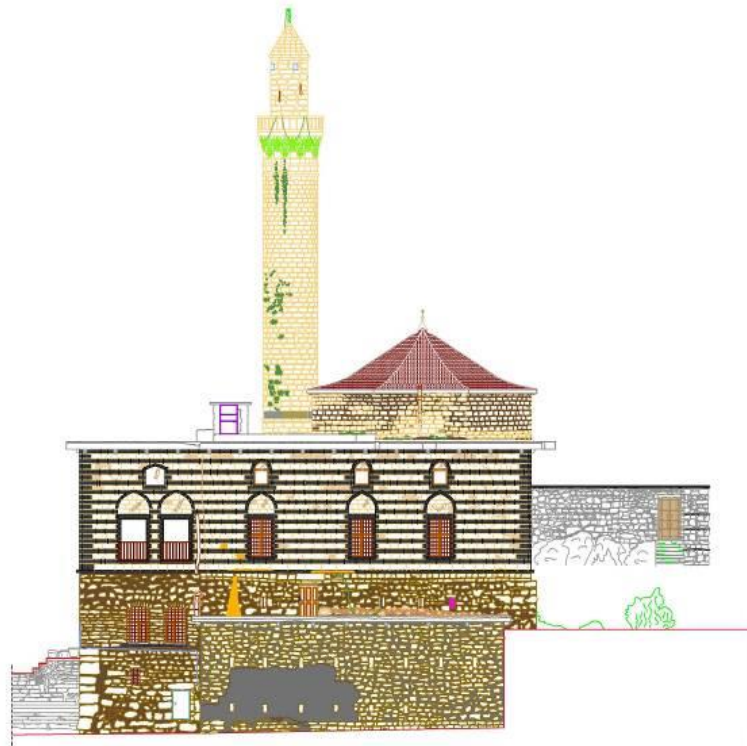
Çizim:8 - Hazro Ulu Camii'nin Batı Cephe Görünüşü Ölçek: 1/50 (Vakıflar Bölge Müdürlüğü Arşivinden).
