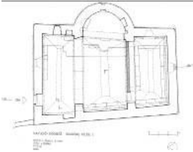
Çiz. 18) Plan.
