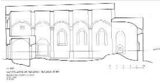
Çiz. 6) Boyuna Kesit.
