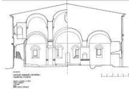
Çiz. 20) Enine Kesit.
