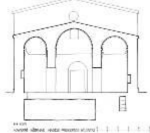
Çiz. 3) Enine Kesit.
