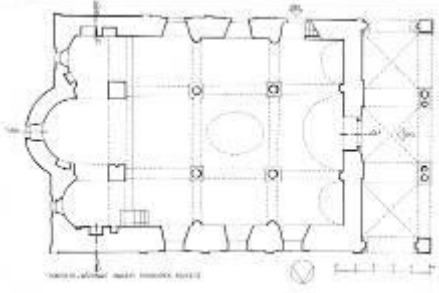
Çiz. 1) Plan.
