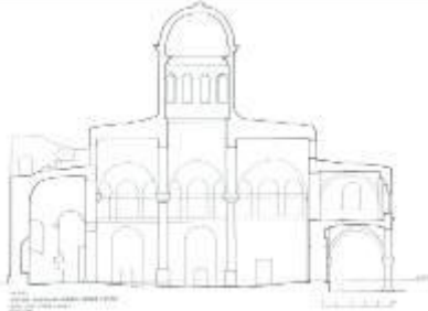
Çiz. 22) Boyuna Kesit.
