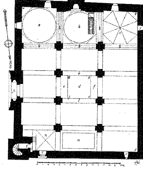
Çizim 2. Niğde Alaeddin Camii, plan (A. Gabriel, 1931)
