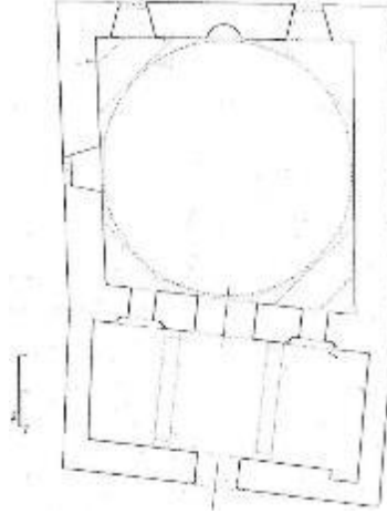
Çizim 1. Konya Beşarebey Mescidi, plan (Y. Önge, Vakıflar Genel Müdürlüğü Arşivi)
