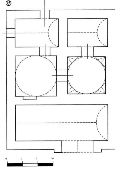
Çiz. 1. Taraklı Yunus Paşa Hamamı (Y.ÇETİN)
