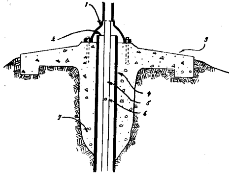
ŞEKİL 3. Delme suretile yapılmış kuyu konstrüksiyond
