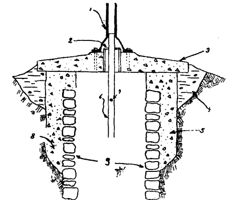
ŞEKİL 2. Kazma suretile yapılmış eski bir kuyu ağzının yeniden inşası metodu
