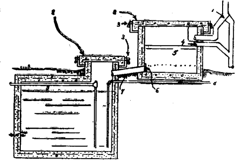
ŞEKİL 5. Hazneye gelen suyu süzmeye mahsus kum filtre tertibatı
