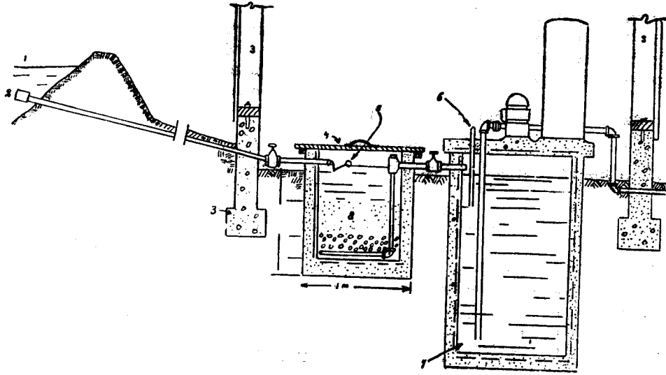
ŞEKİL 6. Toprak yüzünden akan sulardan istifade etmeyi temin eden tesisat
