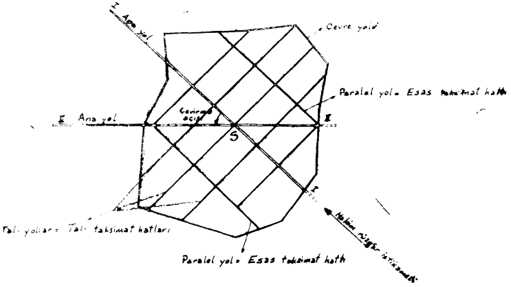
Resim 2 . Düz ve yayvan arazide orman iç taksimat şebekesiyle yol şebekesinin birbirine intibaki.
