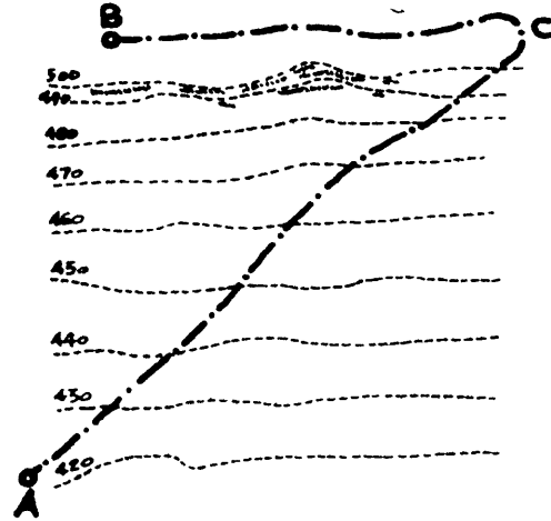
Resim 3 . Yamaç üzerinde diyagonal çıkış.
