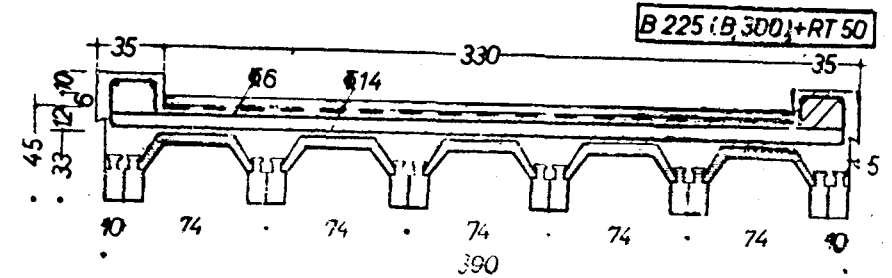
Şekil 9. Hazır betonarme kirişli köprü enkesiti
