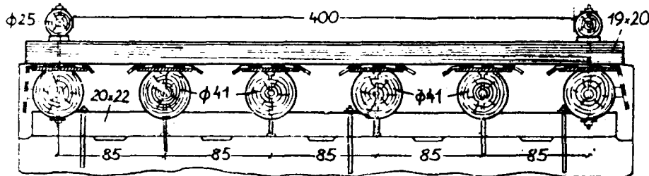
Şekil 4. Ahşap yuvarlak kiriş ve kalas tabliyeli köprü en kesiti
