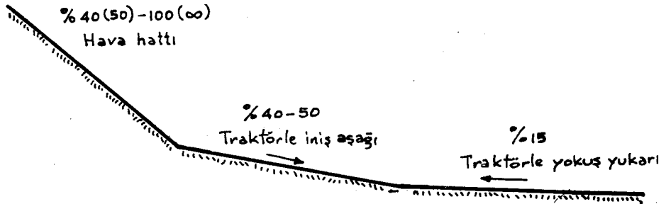
Şekil 3. Çeşitli nakliyat şekillerinin uygulanacağı eğim sınırları
