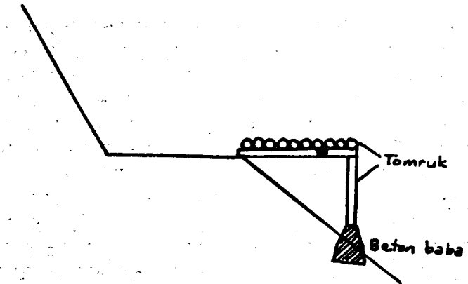
Şekil 16. Dik yamaçlarda yolun alt tarafından hazırlanan beton ayaklar üzerine tomruklarla kurulan çalışma yeri kesiti
