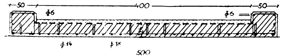
Şekil 6. Torçelik betonarme tabliyeli köprü enkesiti
