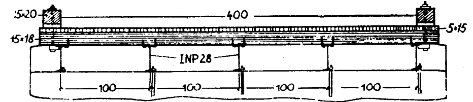
Şekil 5. Çelik kiriş ve ahşap tabliyeli köprü enkesiti
