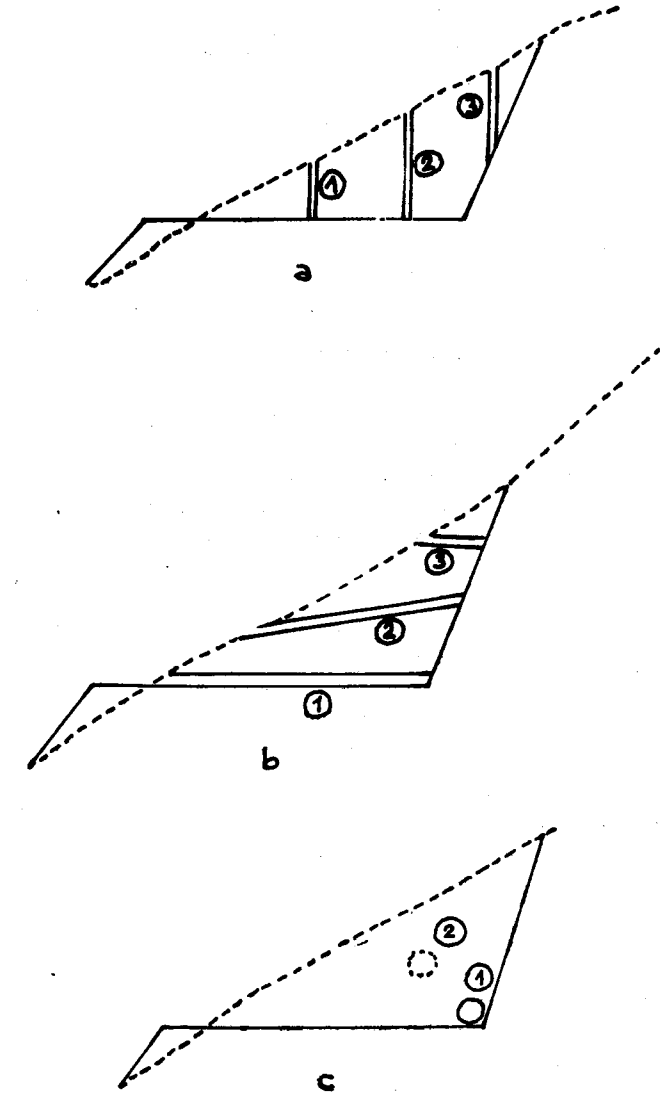
Şekil 14. Yol inşaatında yapılacak kaya hafriyatında lâğım deliği açma metodları
