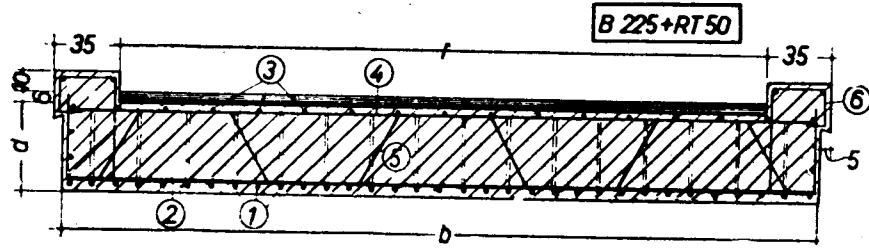
Şekil 7. Nervürlü torçelik betonarme tabliyeli köprü enkesiti
