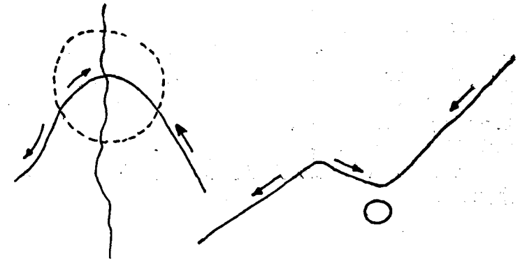
Şekil 13. Yamaç yollarının mecraları katettiği yerlerde aksi meyil uygulayarak suların yola zarar vermeden akıtılması.
