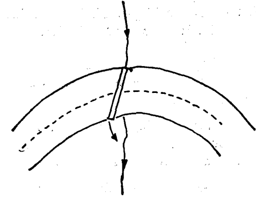
Şekil 11. Tabii mecraya meylinin % 15 i aşması halinde büz istikametinin değiştiği
