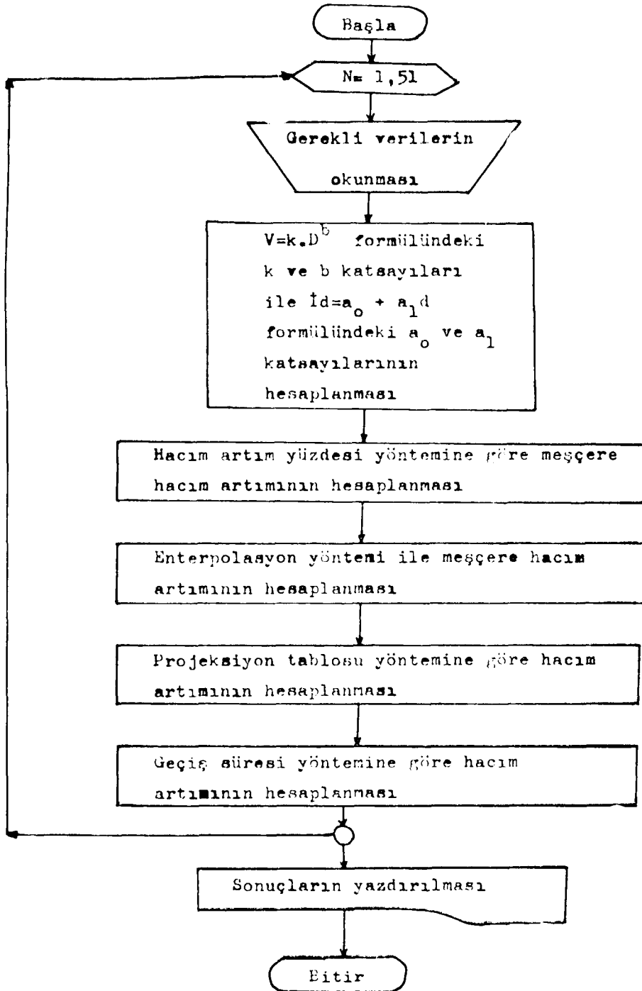
Şekil 1. ORMAN isimli bilgisayar programının genel akış diyagramı.
