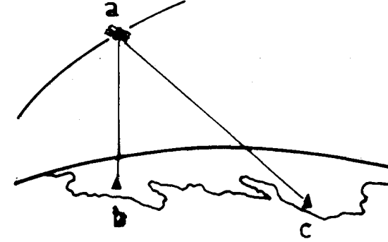
Şekil 7. Koordinatları bilinen bir yer istasyonundan ve uydudan yararlanarak, yeni bir istasyonun koordinatlarının nasıl bulunduğunu gösteren şekil. b istasyonunun koordinatları bilinmektedir. a noktasında bulunan uydunun ve b, c noktalarındaki istasyonların gönderdiği sinyallerden yararlanılarak, önce a noktasının, daha sonra da c noktasının koordinatları bulunabilmektedir. Bu yöntem, uydunun yörüngesinde giderken, meydana gelen küçük sapmalardan etkilenmez ve c noktasının koordinatlarının daha duyarlı şekilde bulunmasına olanak sağlar.
