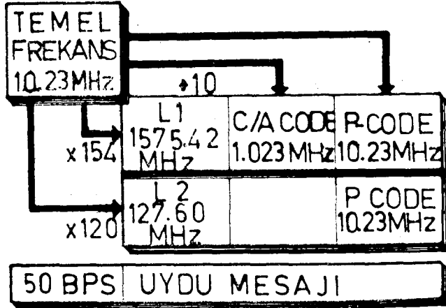
Şekil 3. Şekil 1'deki uyduların, sinyal gönderirken kullandıkları dalgaların frekanslarını gösteren şema. Uydularda üretilen dalgaların temel frekansları 10,23 m Hz dir. Sol yukardaki kare bu dalgaları göstermektedir. Temel frekansların 154 katı L 1 dalgalarını, 120 katı L 2 dalgalarını oluşturmaktadır. Temel Frekansların 0,1'i «Yaklaşık Yöntem» de kullanılan C/A kod'lu dalgaları vermektedir. «Duyarlı Yöntem» de kullanılan P kod'lu dalgaların frekansları, Temel Frekansın aynıdır. Temel Frekansla üretilen dalgalarından ayrı olarak, uydular 1/50 saniye aralıklı özel sinyaller ve mesajlar göndermektedirler.
