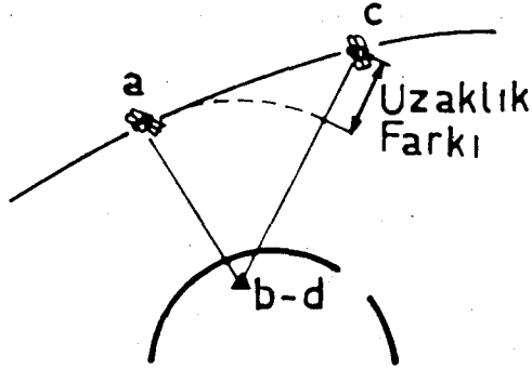
Şekil 6. Uydunun yer istasyonu arasındaki uzaklığın, değişimini gösteren şekil. Başlangıçta uydunun a noktasında, yer istasyonu b noktasındadır, aralarındaki uzaklık ab'dir. Biraz sonra uydunun c noktasına gelmesiyle, yer istasyonu b noktasından c noktasına olan uzaklık bc olur. Bu durumda, yer istasyonu b noktasından c noktasına olan uzaklık, başlangıçta olan ab'den daha büyüktür. Şekil, bu uzaklık farkını göstermektedir. Ayrıca, yer istasyonu b noktasından c noktasına olan uzaklık, başlangıçta olan ab'den daha büyüktür. Şekil, bu uzaklık farkını göstermektedir.
