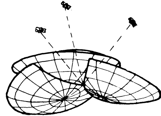
Şekil 4. Uzayda, Önden Kestirme (İlerden Kestirme) yönteminin nasıl uygulandığını gösteren yekil. GPS yönteminde, yani noktaların dünyadaki yerlerinin bulunması yönteminde, uydu ile yer istasyonu (algılayıcı alet) arasındaki uzaklık, çok duyarlı şekilde ölçülmektedir. Uzaydaki bir noktadan (uydudan) eşit uzaklıkta bulunan noktaların geometrik yeri bir küre yüzeyidir. Şekildeki 3 uydunun yer istasyonundan uzaklıkları ölçülmüş ve her biri için bir küre yüzeyi çizilmiş olduğu görülmektedir. 3 küre yüzeyinin kesiştiği nokta, yer istasyonunun, uydulara göre bulunduğu noktadır.
