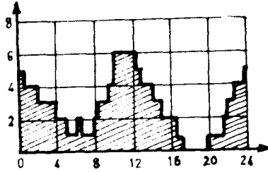
Şekil 2. Şekil 1'de görülen uydular, tamamlandığı ve çalışmaya başladıklarında, dünyanın çeşitli noktalarında, hangi uyduların hangi saatlerde geçeceği araştırılmaktadır. Yukardaki şekil İsviçre'nin Heerbrugg şehriden 20 Haziran 1985 günü geçen uydular ve geçiş saatlerini göstermektedir. Buradaki grafik, bu gün dolaşan uydu sayısına göre çizilmiştir. Yatay eksen uyduların geçiş saatlerini, dikey ekseninde sayılarını göstermektedir.
