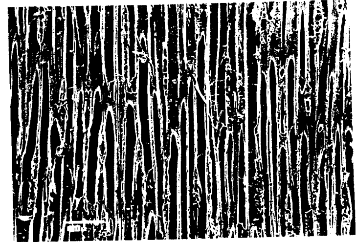
Şekil 4: Pinus nigra var. pallasiana odunu teğet kesiti (X150) Figure 4: Tangential section of Pinus nigra var. pallasiana (X150)
