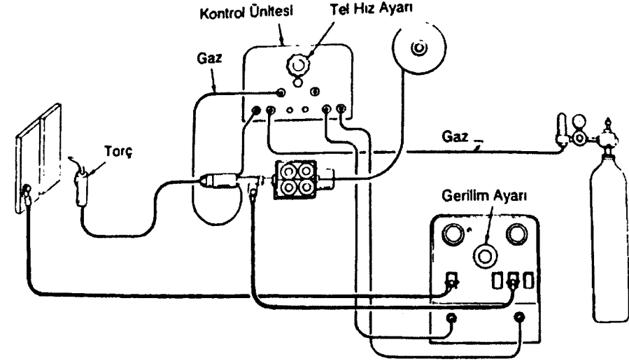
Şekil 3. MIG/MAG kaynak donanımı blok şeması (Ertürk, 1987).
