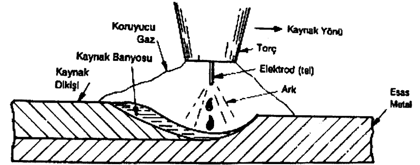
Şekil 2. MIG kaynak metodunda ark bölgesi (Tülbentçi, 1990).
