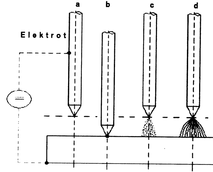
Şekil 1. Ark oluşumu: a) elektrot iş parçasına henüz değmiyor (devre açık), b) elektrot iş parçasına değiyor (devre kapalı), c) iş parçası ısıyor, metal buharları oluşuyor ve havaya karışıyor (hava iletken hale geliyor), elektrot uygun yüksekliğe geri çekiliyor ve d) parlak ışıklı ark oluşuyor (Matthes ve Richter, 2003).
