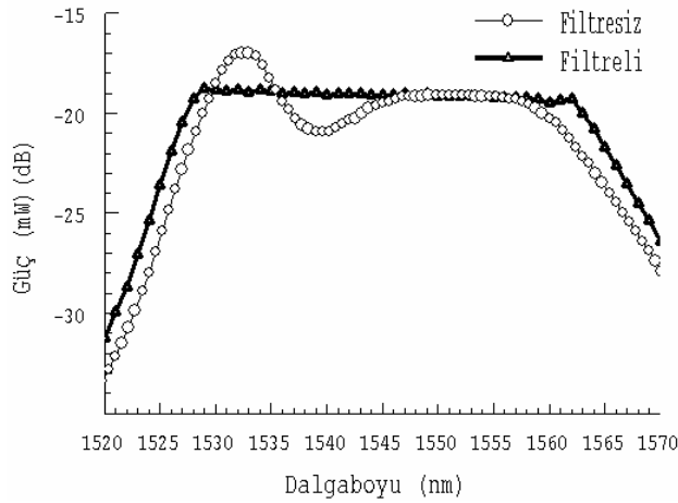
Şekil 6. İki aşamalı EKFY'de filtrenin kullanıldığı ve kullanılmadığı durumlardaki ASE spektrumu
