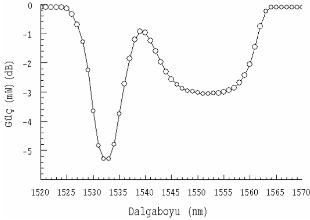
Şekil 5. Optimize edilen filtrenin iletim spektrumu
