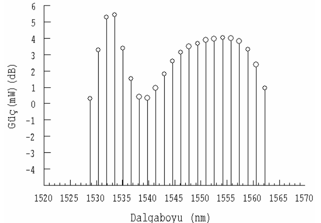
Şekil 3. Filtresiz iki aşamalı EKFY'de giriş sinyaline karşılık çıkış sinyali. (a) Giriş sinyali, (b) Çıkış sinyali
