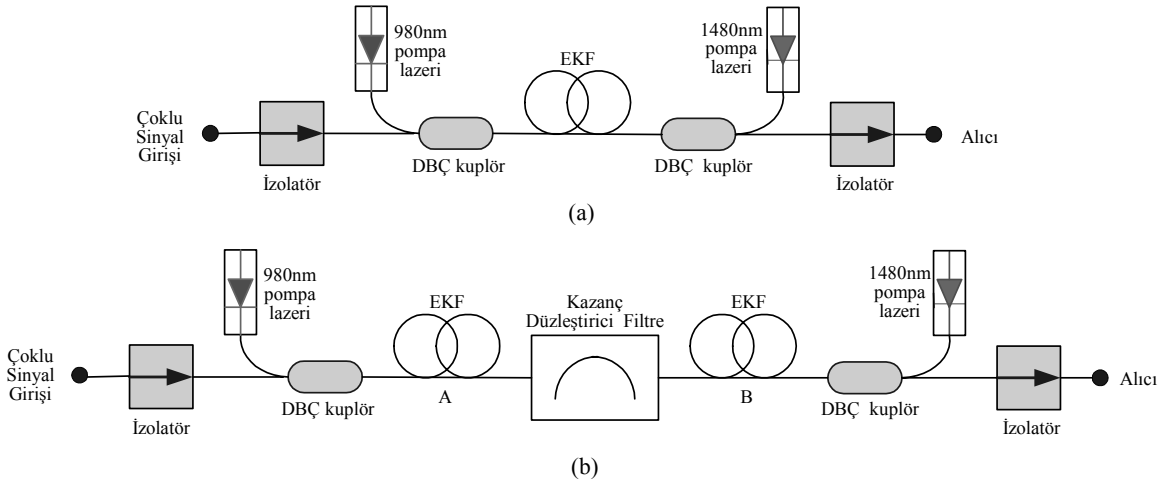
Şekil 2. Kazanç düzeltirici filtre ile iki aşamalı EKFY'nin kazanç optimizasyonu düzeni, (a) Filtresiz düzenek, (b) Filtreli düzenek
