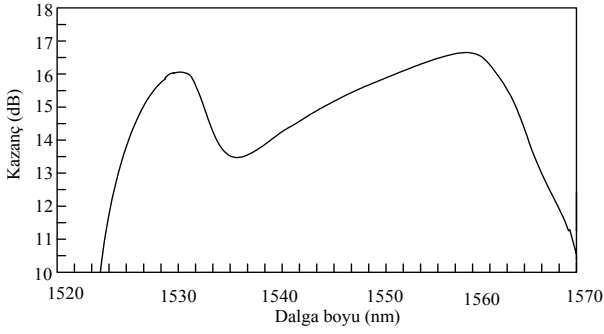
Şekil 1. EKFY'nin dalga boyuna bağlı kazanç spektrumu
