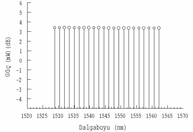
Şekil 4. Filtre kullanılan iki aşamalı EKFY'nin çıkış sinyalleri
